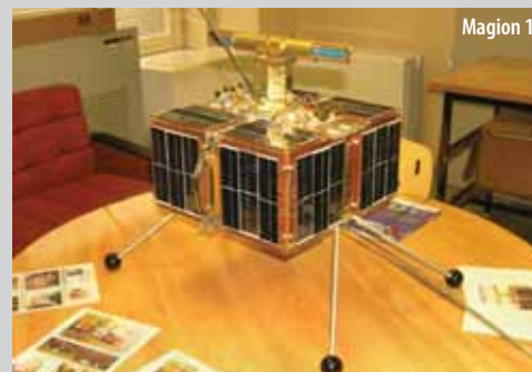
Magion 1
