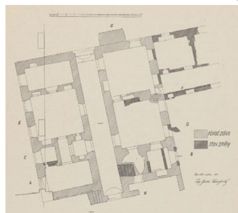
Půdorys přízemí Kurzovského domu. Podle R. Hlubinky
