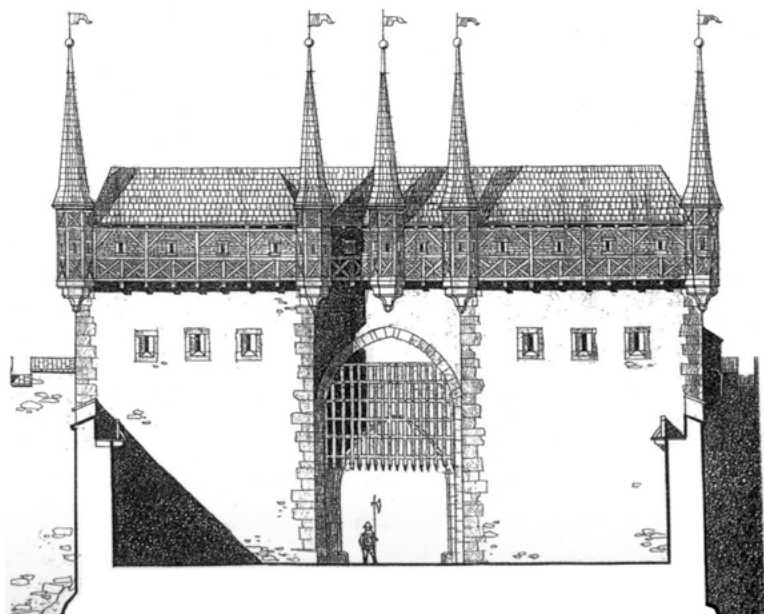
Kresebná rekonstrukce brány v pohledu (podle Františka Kašičky)
