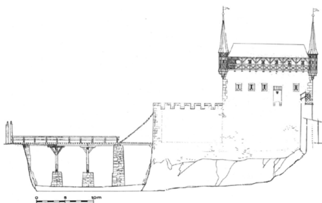
Rekonstrukce pravděpodobné podoby brány s předbranním a padacím mostem (podle Františka Kašičky)
