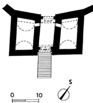
Kresebná rekonstrukce brány v půdorysu (podle Františka Kašičky)
