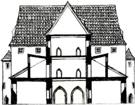
Příčný řez kotci na Havelském tržišti. Dnešní ulice V Kotcích bývala převýšenou středovou halou, dnešní zástavba podél ulice zaujala místo bočních lodí. Podle Viléma Lorence
