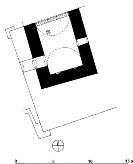
Náčrt situace jedné prostory gotického sklepa pod sýpkou. Podle L. Jindřicha kreslil Jiří Úlovce.
