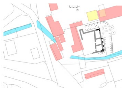
Rekonstrukce podoby mladší z dubčských tvrzí. Černě stávající dochované zdivo, šedě rekonstruovaný průběh zdiva na základě geofyzikálního a stavebně-historického průzkumu. Modře průběh Říčanského potoka, červeně zděná zástavba, žlutě dřevěná zástavba (vše podle mapy stabilního katastru okolo roku 1841). Oranžově půdorys sklepů starší dubčské tvrze. Podle Vojtěcha Kašpara.
