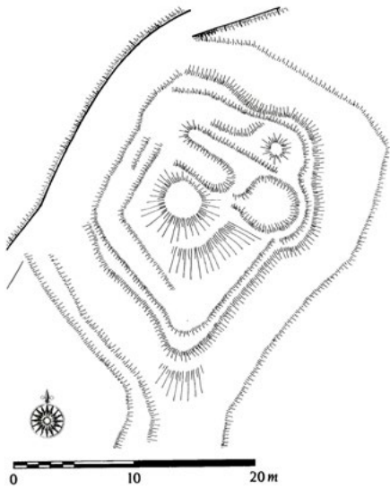
Náčrt situace tvrzště. Podle zaměření J. Jindřicha kreslil J. Úlovec.
