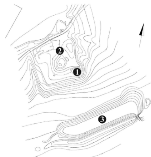
Vrstevnicový plán tvrziště Slavětice. 1 – pravděpodobný relikv věže; 2 – pravděpodobný pozůstatek obytné budovy; 3 – umělá vodní nádrž – příkop. Podle P. a J. Kárníka
