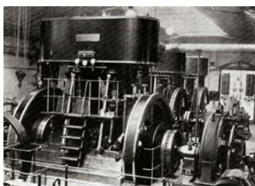
Interiér elektrárny
