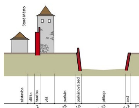
Ideální řez středověkým opevněním Starého Města. Podle P. Juřiny, 2009
