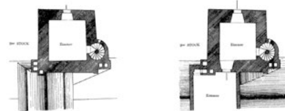
Zaměření věže z roku 1893. Půdorys druhého a třetího patra a pohled od jihu a západu. Podle A. Wiehla.
